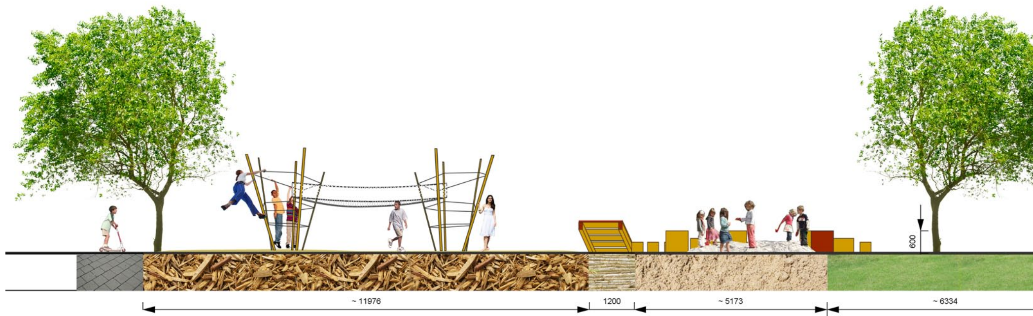
Doorsnede BB
