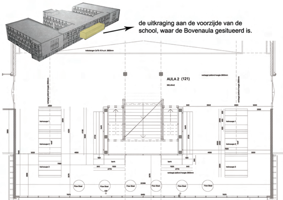
Plattegrond Definitief Ontwerp Bovenaula
